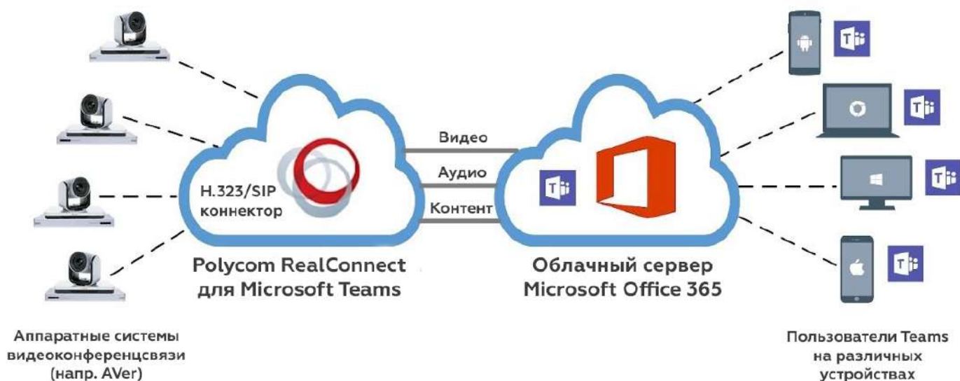
Визуализация схемы работы шлюза на примере RealConnect
