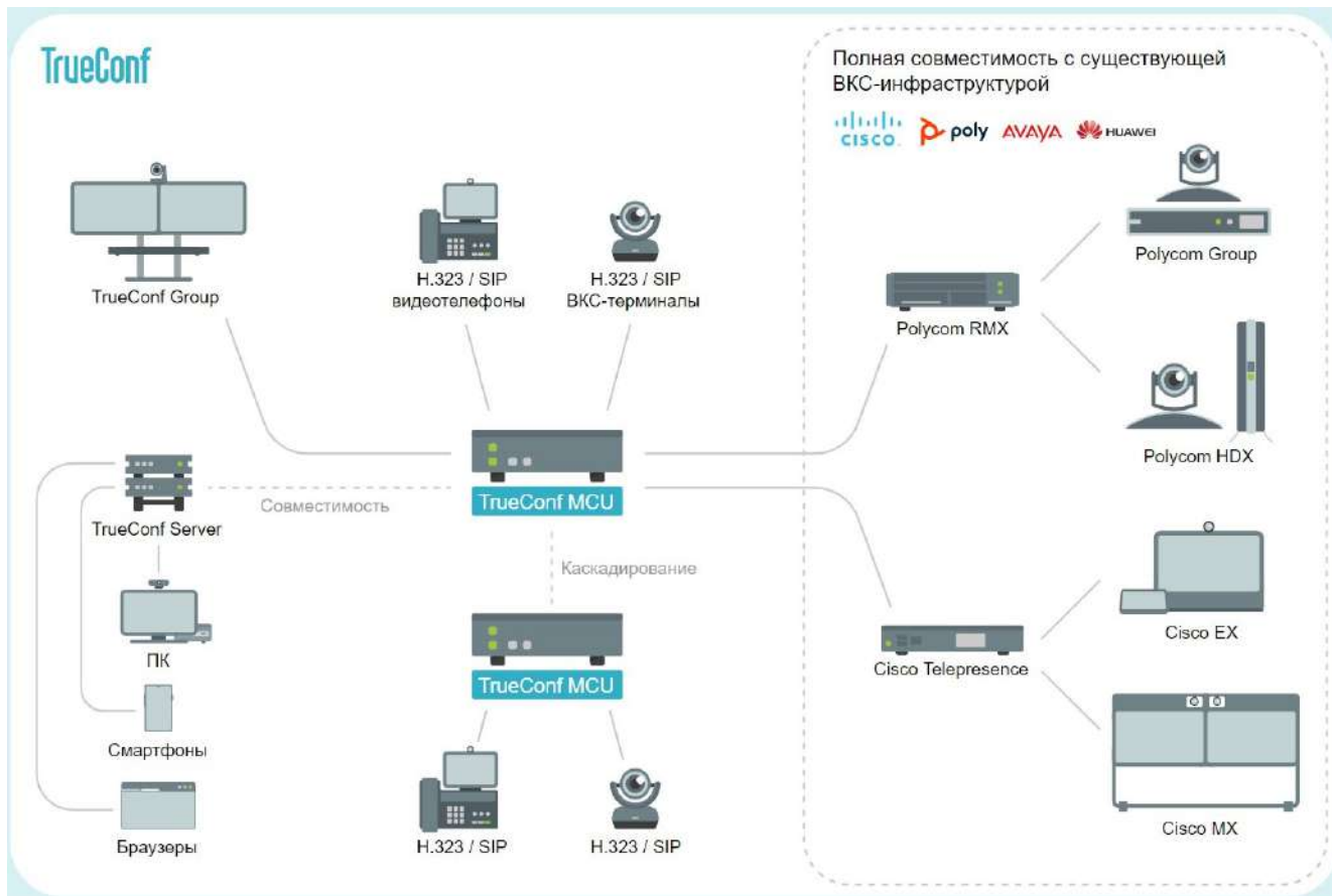
Пример крупномасштабной структуры сети видеоконференцсвязи от TrueConf, собранной из множества различных брендов. С каждым из которых совместим и AVer. На схеме он может находиться в "H.323/SIP ВКС-терминал", либо заменить любое брендовое устройство.
