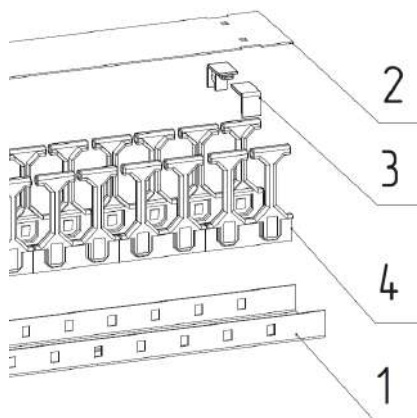
Конструкция нового органайзера TLK
